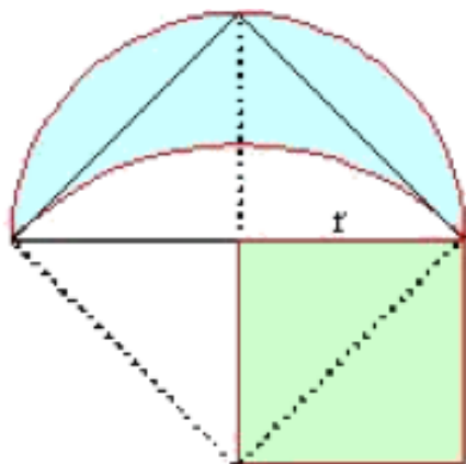
Figura #3: Cuadratura de una lúnula propuesta por Hipócrates de Quíos.
