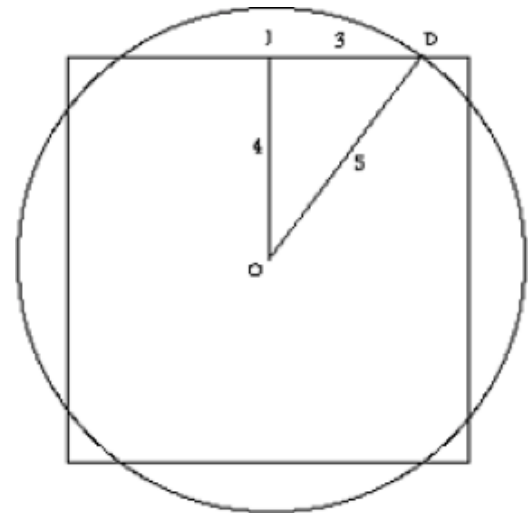
Figura #1: El círculo y el cuadrado.
