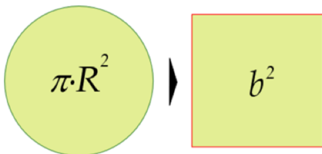
Figura #2: Formulas del área del círculo y el cuadrado.
