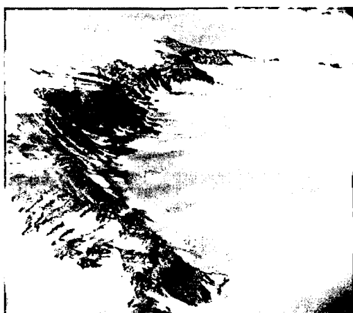
Vista aérea de las grietas antárticas tomadas por la expedición alemana de 1938-39.
